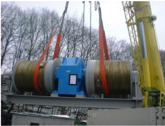
Seilwinden für Gefäßhubsystem
